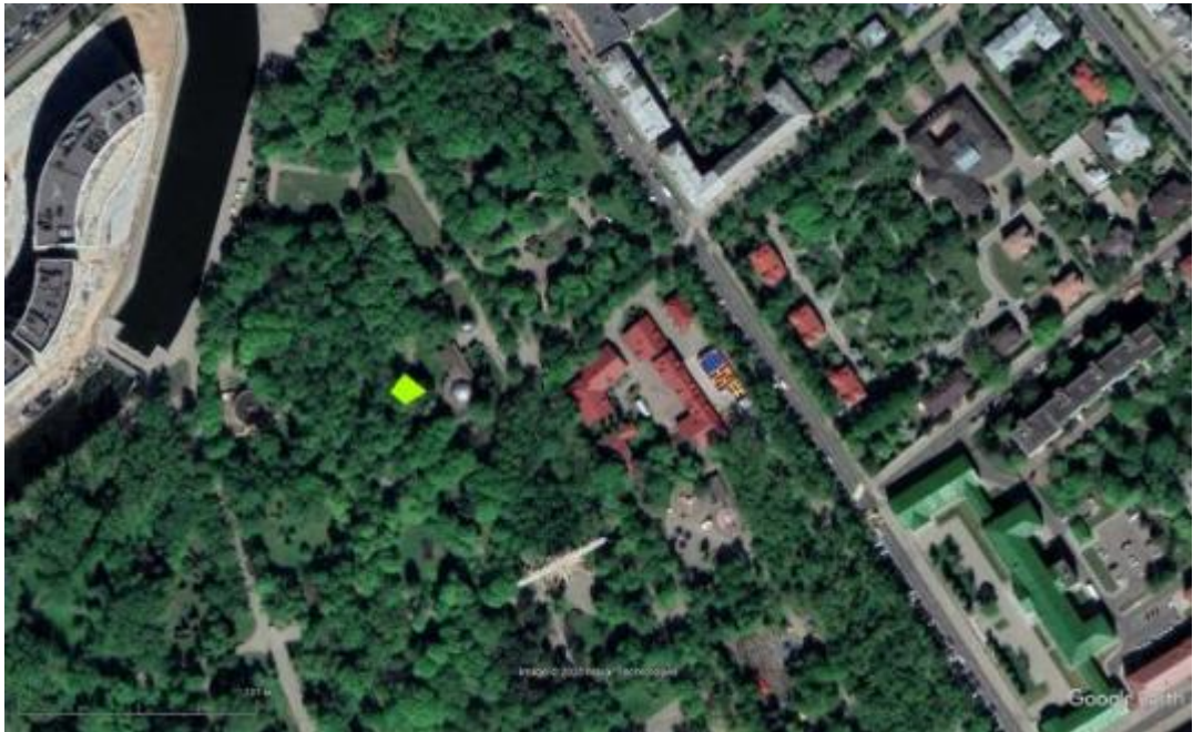
Рисунок 7 – Ситуационная схема памятника природы местного значения «Липа Губернаторского сада»
