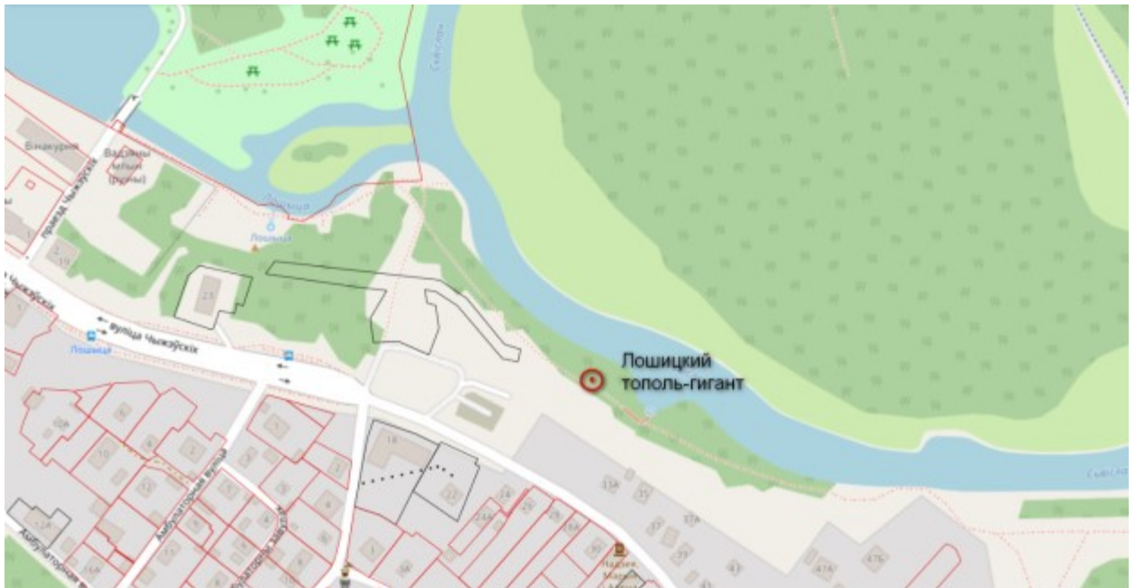
Рисунок 14 – Ситуационная схема резервируемого ботанического памятника природы местного значения «Лошицкий тополь-гигант»
