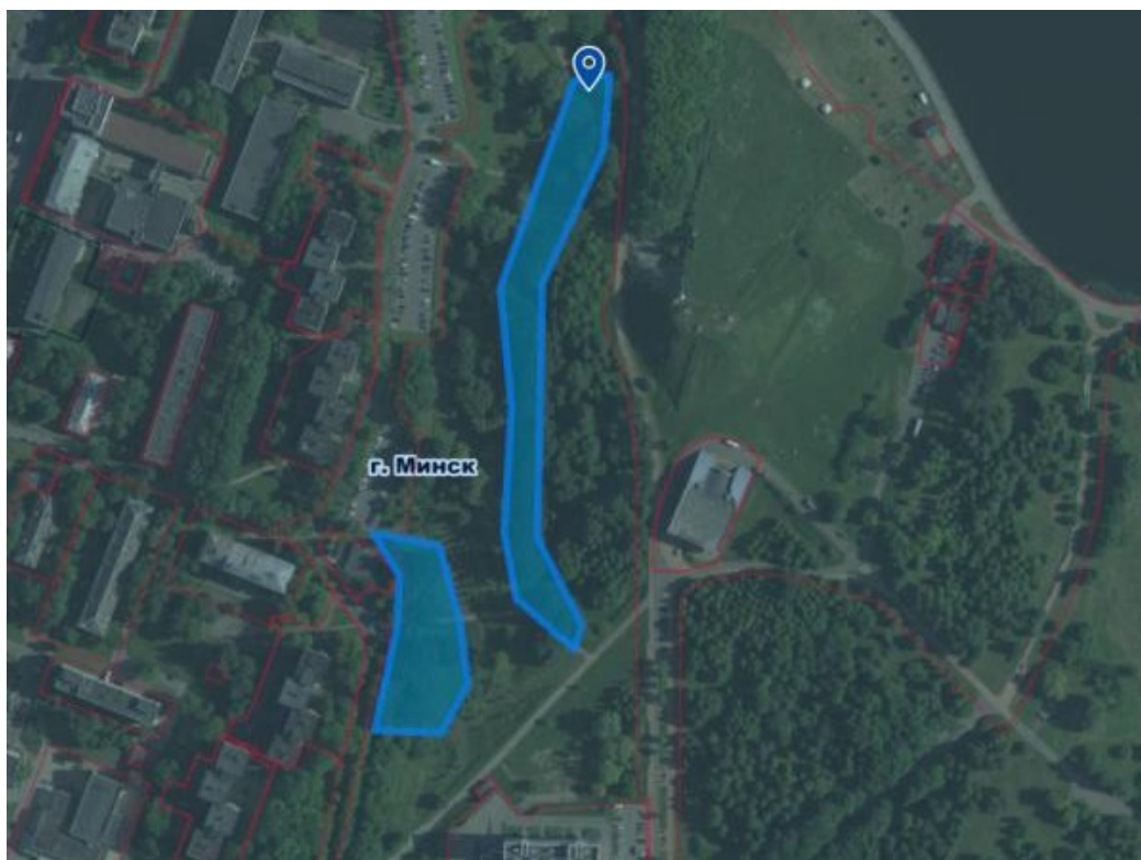
Рисунок 2 – Ситуационная схема памятника природы местного значения «Вековая дубрава парка «Курасовщина»
