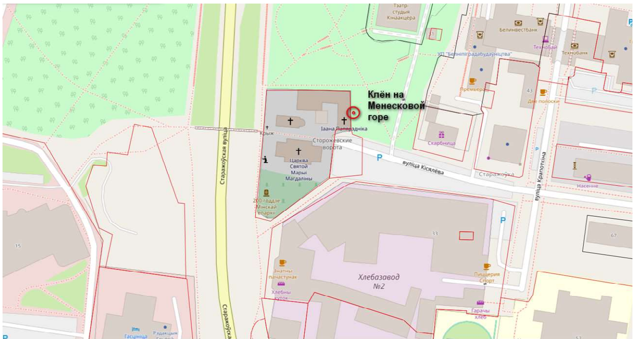
Рисунок 17 – Ситуационная схема резервируемого ботанического памятника природы местного значения «Клен на Менесковой горе»
